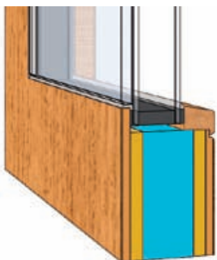
E steklo v ravnini s krilom na zunanji strani
