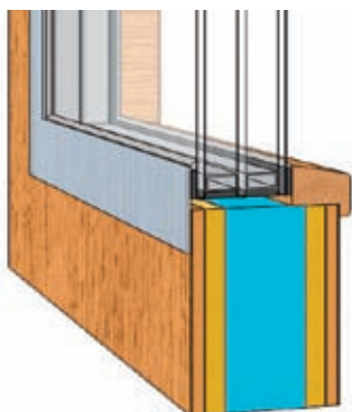
D okvirček iz nerjavečega jekla na zunanji strani
