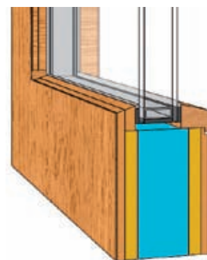
C letvica znotraj zamik stekla 22 mm na zunanji strani
