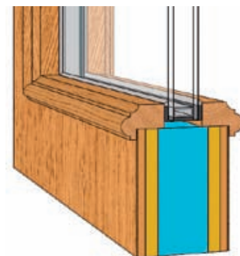
F letvica obojestransko rustikal
